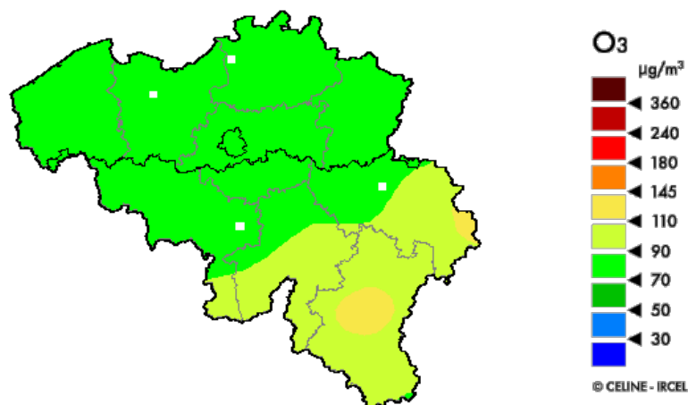
Concentrations horaires maximales prévues pour le samedi 6 juin 2015
